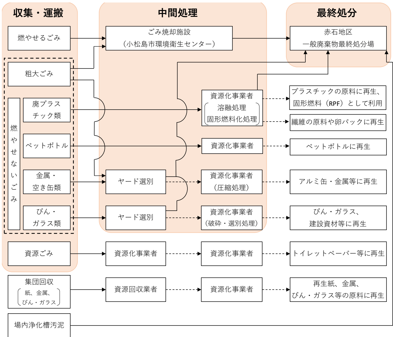
図 3.1 ごみ処理フロー
