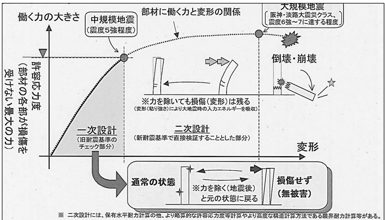
図 5.2 建築基準法の耐震基準の概要
