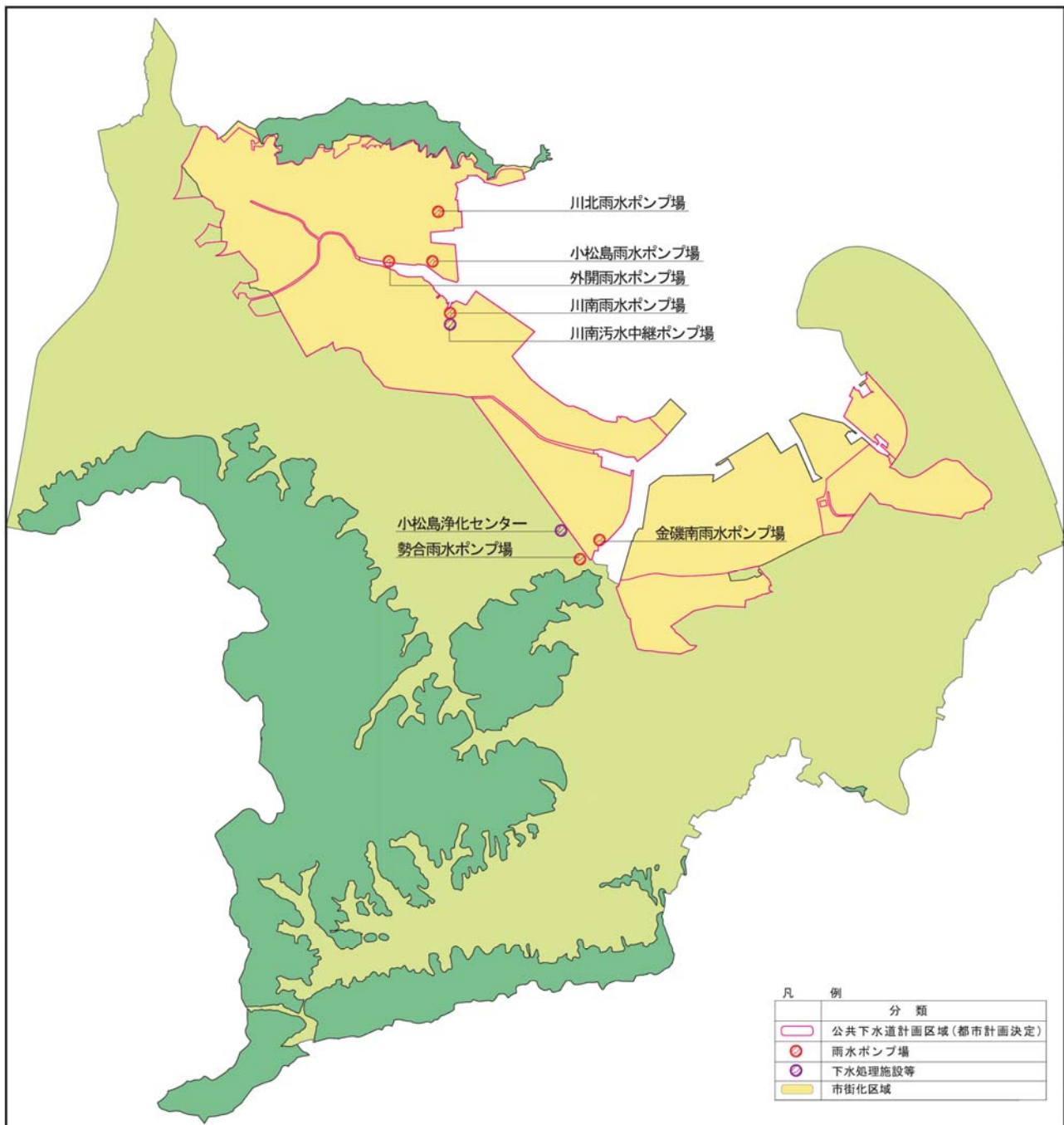
図1-18 下水道の都市計画決定状況図
