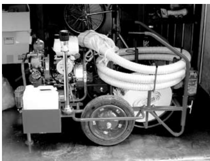
整備された軽可搬消防ポンプ
